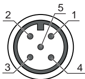
图 6.2: M12 插头 · 5 针 · A 编码
