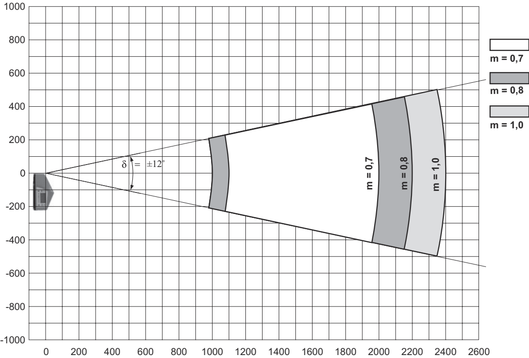
侧面条码阅读曲线
