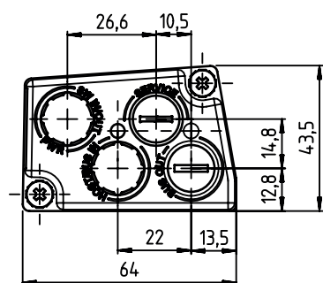
Figura 13.6: Disegno quotato interfaccia di collegamento MS 307
