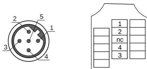
Figura 7.5: Collegamento SSI
