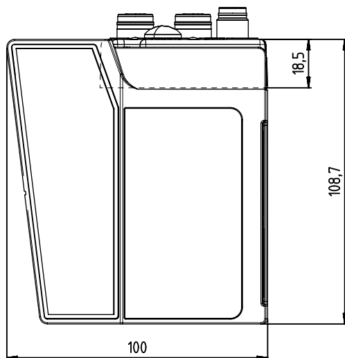
Figura 13.3: Disegno quotato BPS con interfaccia di collegamento MS 307
