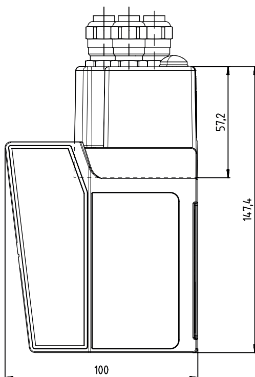
Figura 13.3: Disegno quotato BPS con interfaccia di collegamento MS 307
