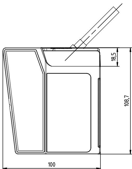
Figura 13.5: Disegno quotato: BPS con interfaccia di collegamento KB 307
