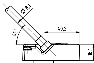
Figura 13.7: Disegno quotato interfaccia di collegamento MK 307
