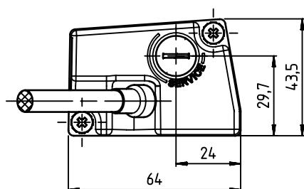
Figura 13.8: Disegno quotato interfaccia di collegamento KB 307
