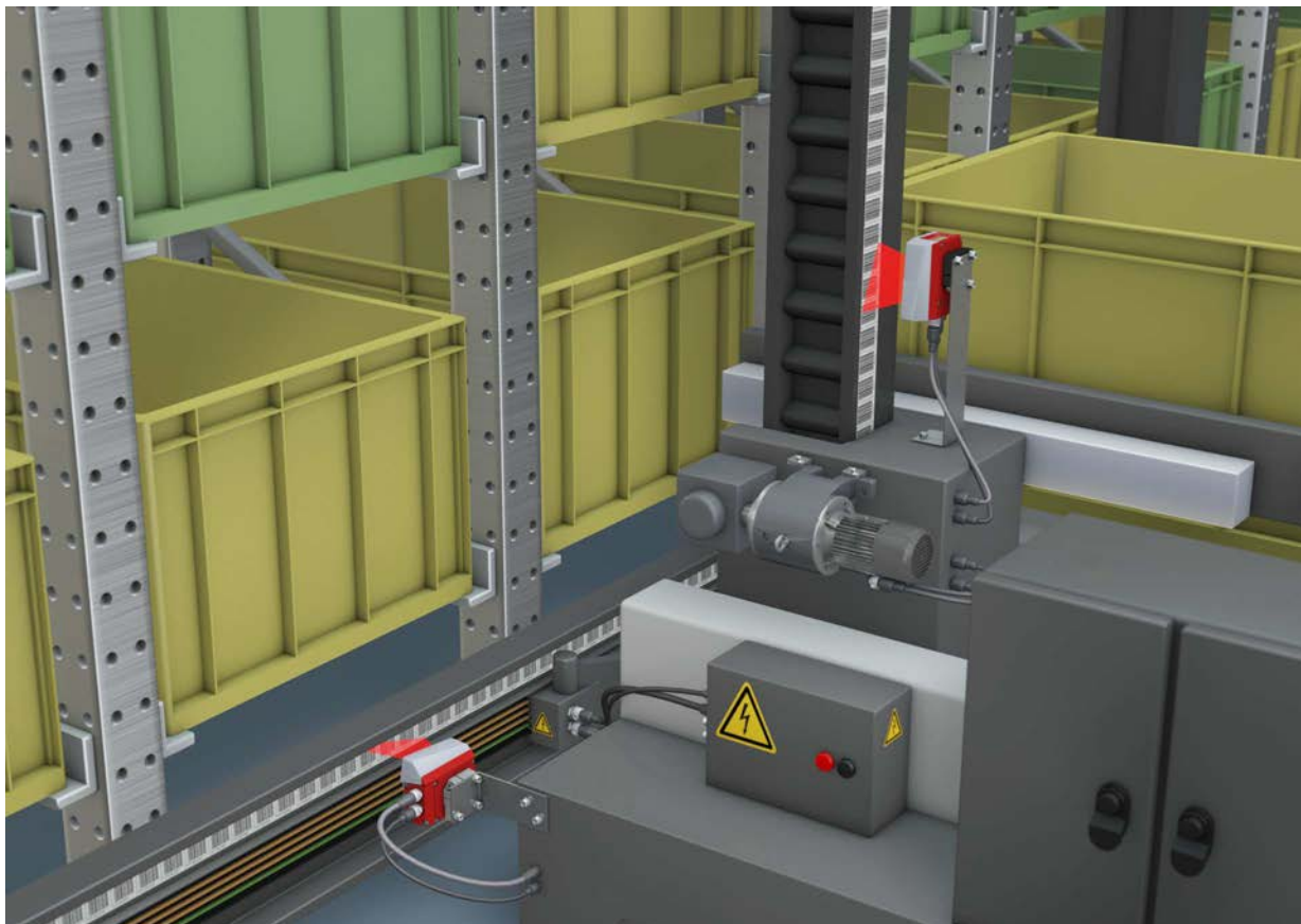
Figura 5.1: Trasloelevatore
