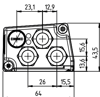
Figura 13.7: Disegno quotato interfaccia di collegamento MK 307
