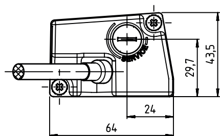
Fig. 13.8: Desenho dimensional tampa de conexão KB 307
