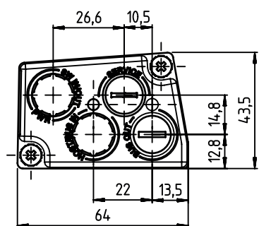
Fig. 13.6: Desenho dimensional tampa de conexão MS 307
