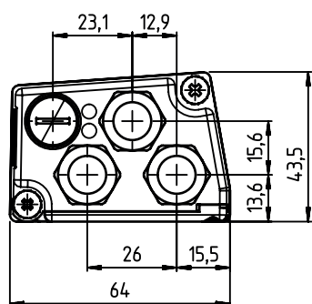
Fig. 13.7: Desenho dimensional tampa de conexão MK 307
