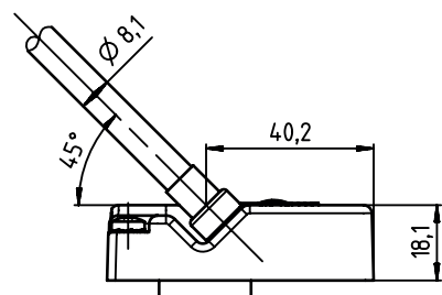
Fig. 13.7: Desenho dimensional tampa de conexão MK 307
