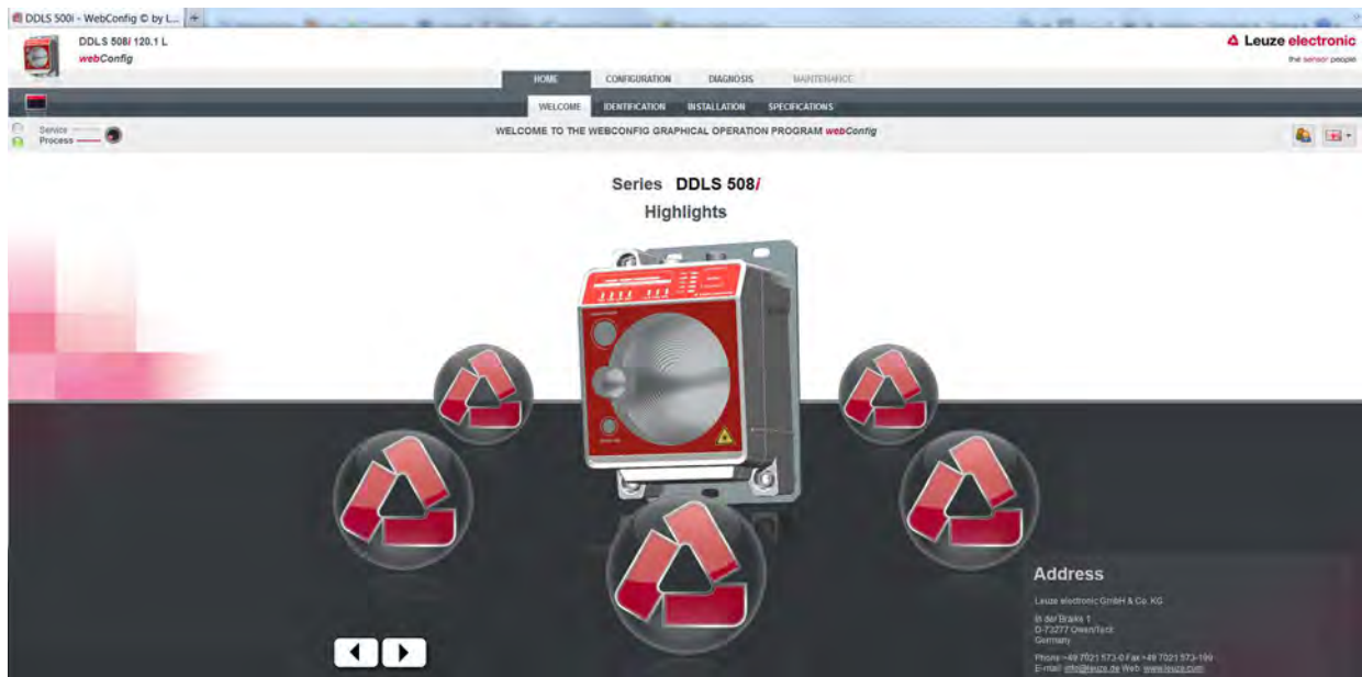
Figura 8.3: Pagina iniziale dello strumento webConfig
