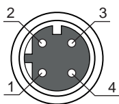
Figura 5.3: Assegnazione dei pin collegamento BUS
