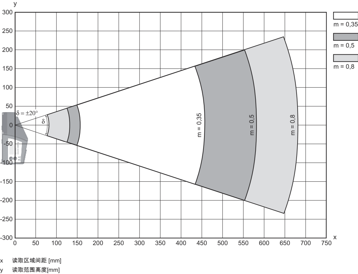
侧面条码阅读曲线
