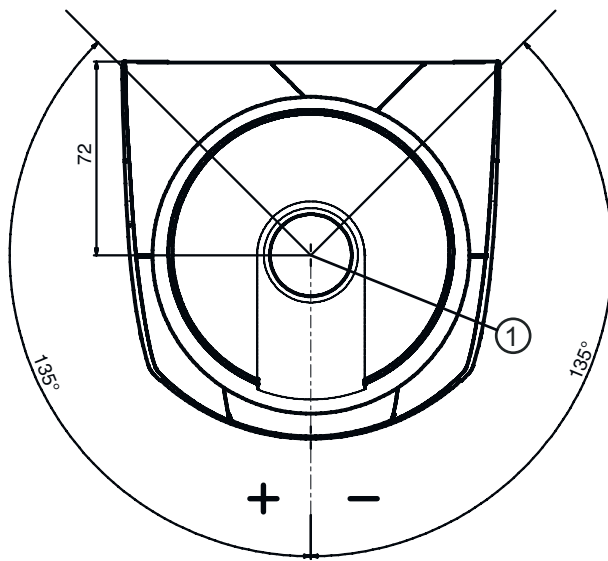
1 거리 측정 기준점 및 보호 필드 반경
