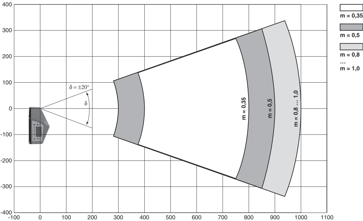
側面の読み取り領域カーブ
