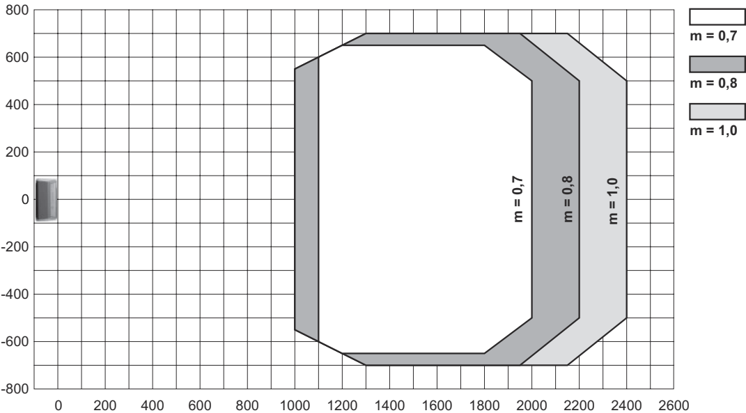
Curva do campo de leitura
