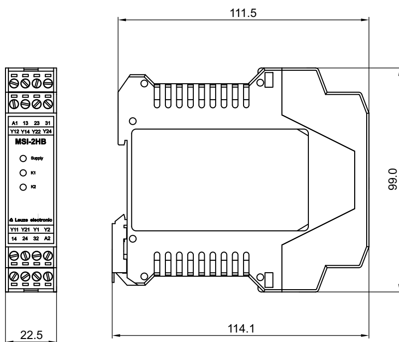
Bild 13.1: Maße MSI-2HB-01
