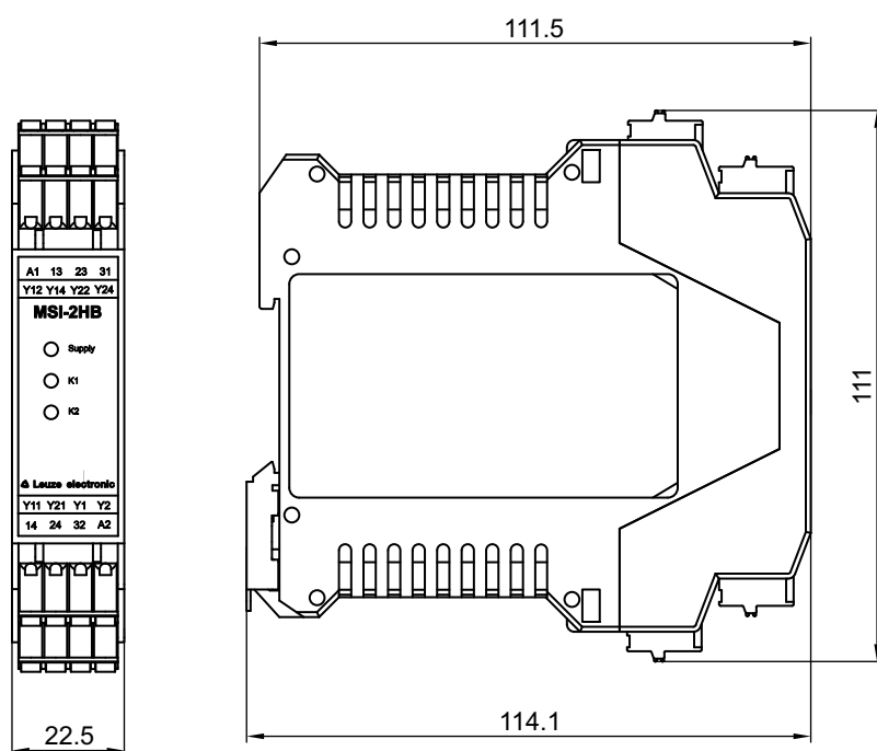
Bild 13.2: Maße MSI-2HB-02
