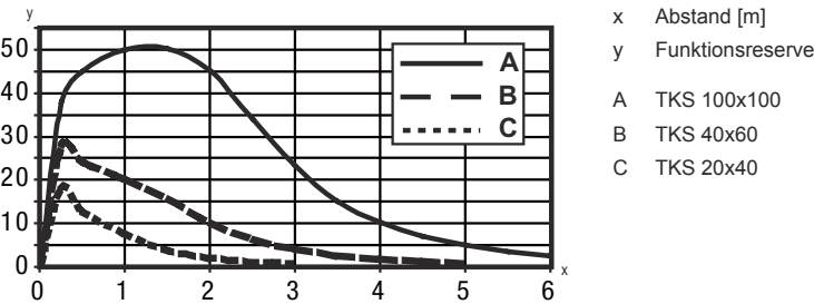
Typ. Funktionsreserve
