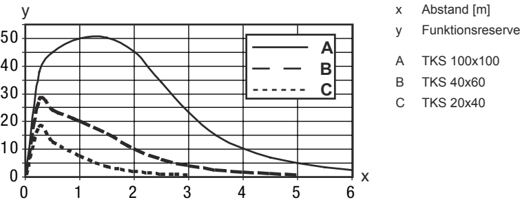
Typ. Funktionsreserve
