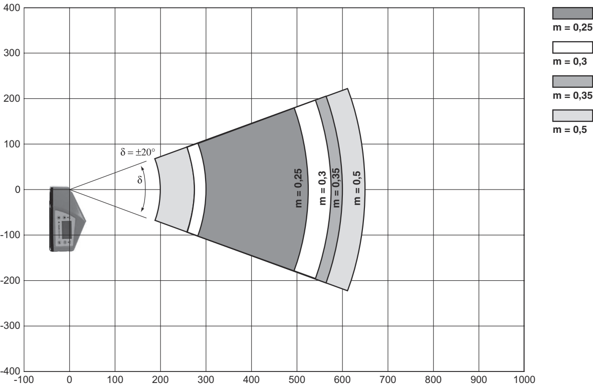
侧面条码阅读曲线
