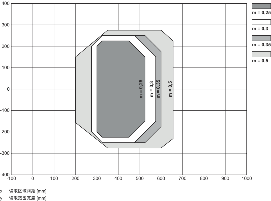
读取区域曲线
